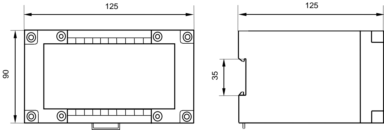
Рисунок В.7 – Габаритные размеры ЦП8507/3 – ЦП8507/6
