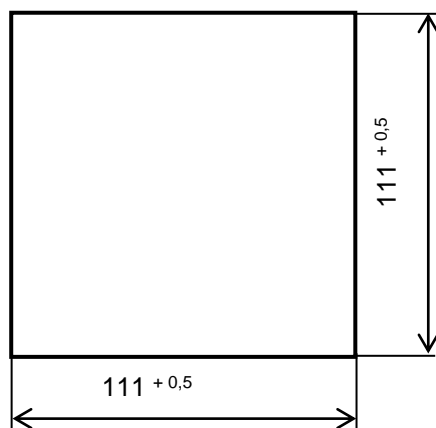
Рисунок В.2 - Габаритные размеры ЦП8507/11 – ЦП8507/14
