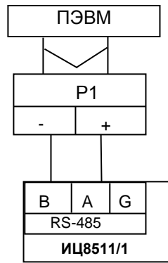
Рисунок Г.8 – Схема подключения ИЦ8511/1, ИЦ8511/2 к ПЭВМ
