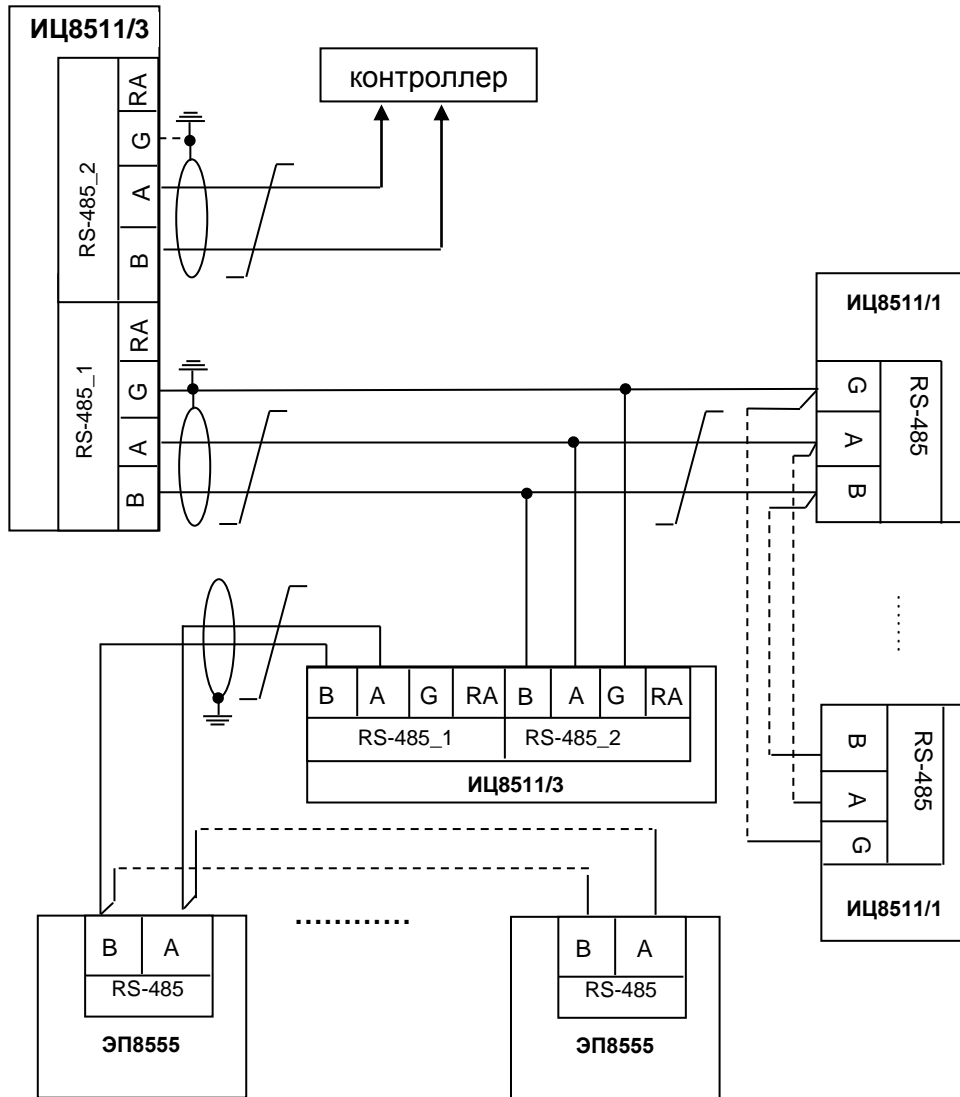
Рисунок Г.7 – Схема подключения индикатора ИЦ8511/3 с приборами и с другими индикаторами ИЦ8511/3 и передачи информации на контроллер и индикаторы ИЦ8511/1
