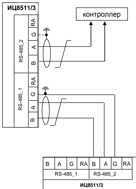
Рисунок Г.5 – Схема подключения индикатора ИЦ8511/3 к ИЦ8511/3 в режиме конфигурации связи и передачи информации на контроллер
