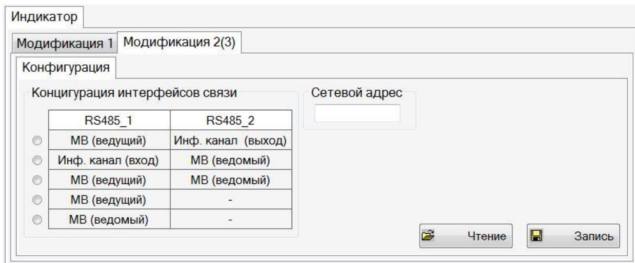
Рисунок 1. – Конфигурации интерфейсов связи в зависимости от выбранных режимов работы ИЦ
