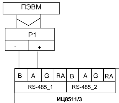
Рисунок Г.9 – Схема подключения ИЦ8511/3 к ПЭВМ
