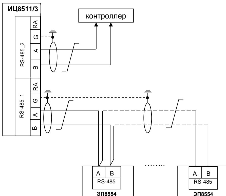
Рисунок Г.6 – Схема подключения индикатора ИЦ8511/3 к приборам и передачи информации на контроллер
