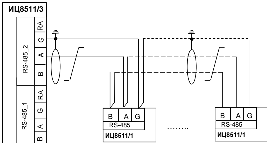
Рисунок Г.2 – Схема подключения индикаторов ИЦ8511/1 к индикатору ИЦ8511/3
